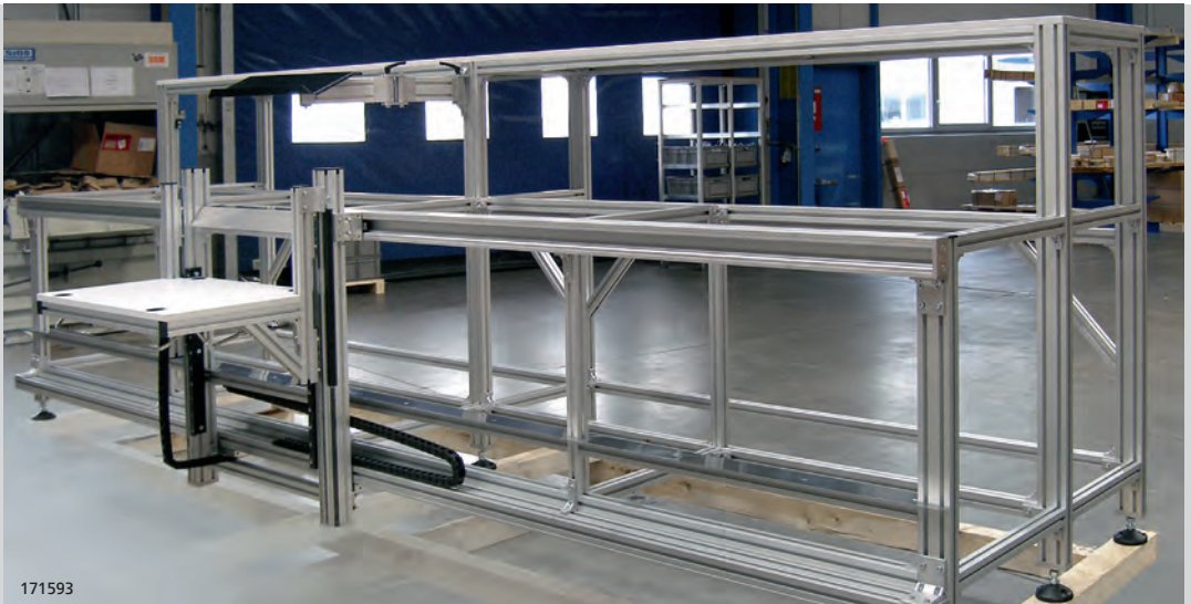
Kommissionier-Regalanlage über Lineareinheiten Horizontal und Vertikal frei verschiebbar
