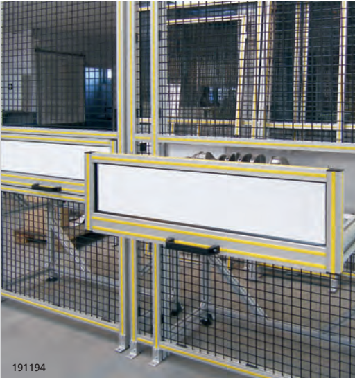
Feld-Lösung inkl. Schublade mit Profilverführungen
