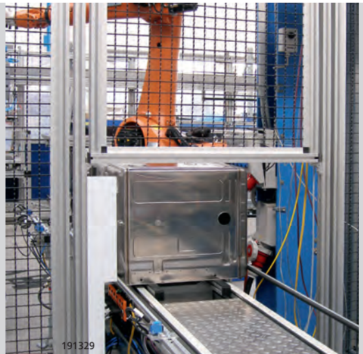
Individuelle Pfosten-Feld-Lösung mit Wellgitter
