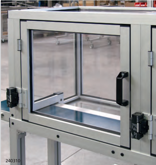
Flügel­tür mit Kugelschnäpper mit Polycarbonat-Füllung
