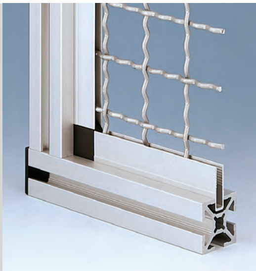
Befestigung für Wellgitter mit Profil mk 2040.60 und Distanzstück
