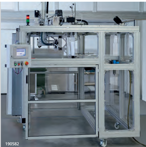
Mobile Schutzhäuser für ein Entnahme- und Stapelmagazin
