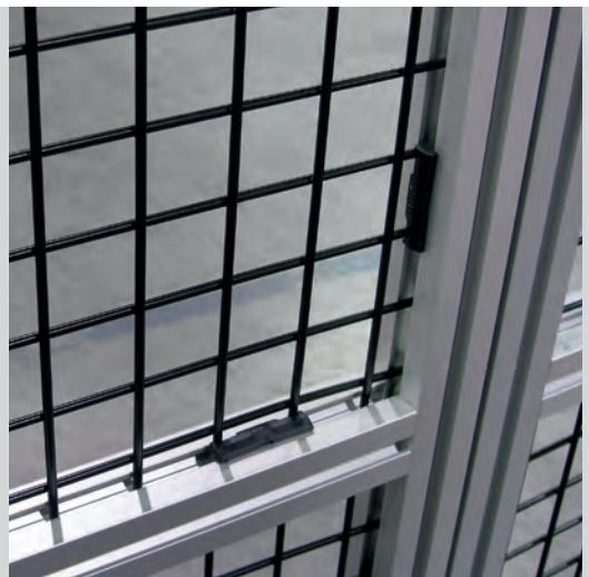
Spannverbinder bei Feldrahmen
