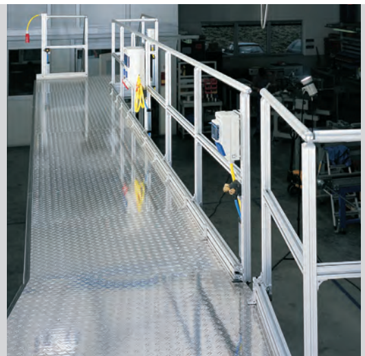
Montagebühne, einseitig durch Geländer abgesichert, Podestboden in Rautenduettblech AL
