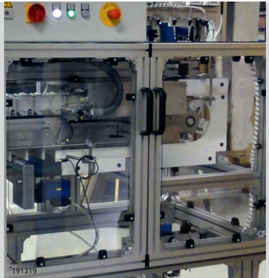
Befestigung mit Scheibenklemmen
