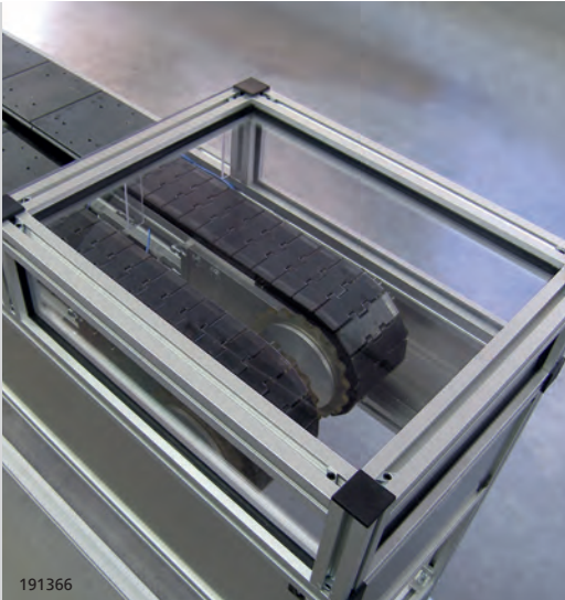
Eingreifschutz aus Flächenelementen Acryl mit Dichtprofil in der Profilvernuth fixiert
