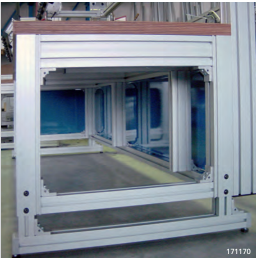
Arbeitstisch schwer mit manueller Höhenverstellung
