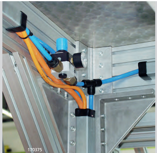
Druckminderventile und Kugelhahn zur Ansteuerung der Luftkissen
