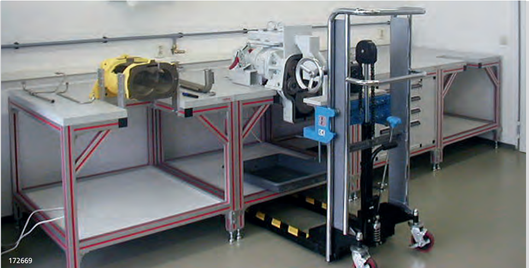
Montagelinie für Pumpen aus Profilerie 50 mit Unterbauschränk und geschlossenen Profilmuten über Verschlussprofil rot
