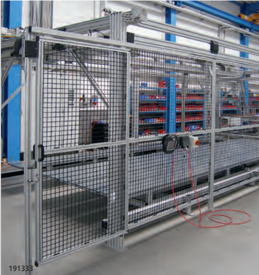
Pfosten-Feld-Lösung mit Schiebetür
