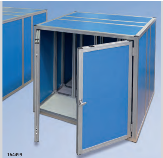
Container mit Doppel-Flügeltür, Drehriegelstangenschloss und Schubriegel
