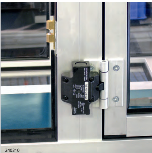
Scharnier-Sicherheitsschalter für drehbare Schutzeinrichtungen, Öffnungswinkel 135°
