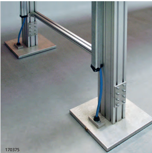
Luftkissen inkl. Zuleitung für den Transport auf ebenem Hallenboden
