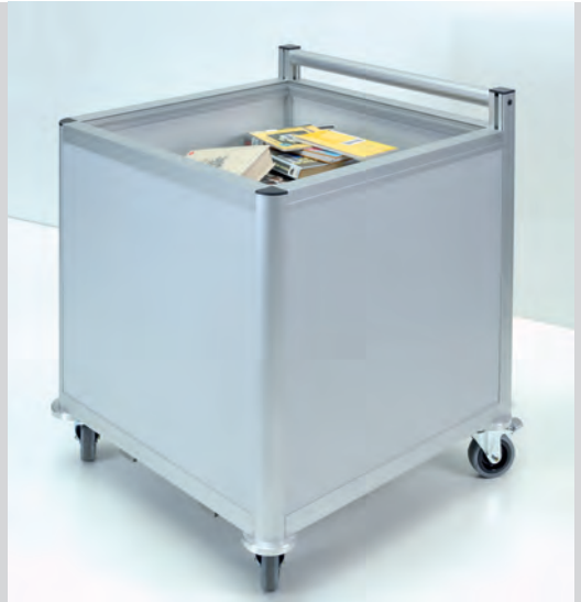
Transportwagen bei dem sich der Federboden bei Gewichtszulage absenkt und bei Entnahme wieder anhebt
