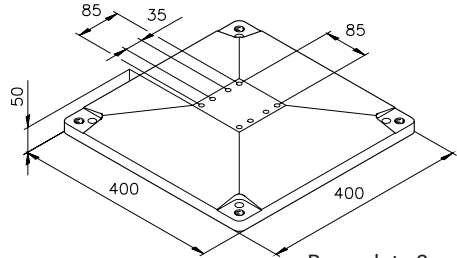
Base plate 2 50.02.0026
