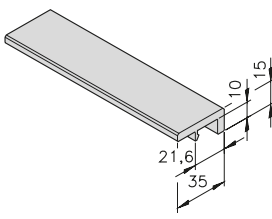
25|40|50|60 Wear strip mk 1040.05 21.05.2000
