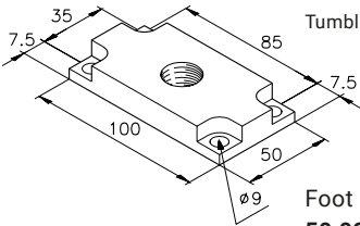
Foot plate B M20 50.02.0004
