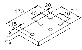
Plate 40/17 50.03.0025
