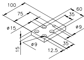
Base plate 1 50.03.0001
