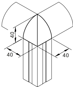
Corner block 42 B46.05.043*
