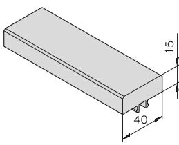
25|40|50|60 Wear strip mk 1040.03 21.03.2000
