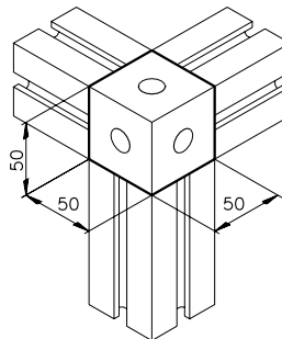
Corner block 4 79.01.0004
